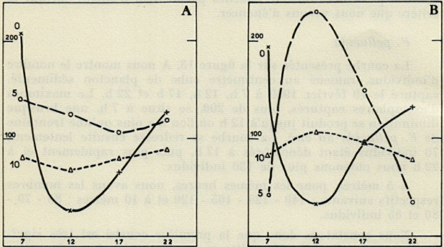
Fig. 13. — A, variation nycthémerale de F. pellucida ; B, variation nycthémerale de O. fusiformis .
